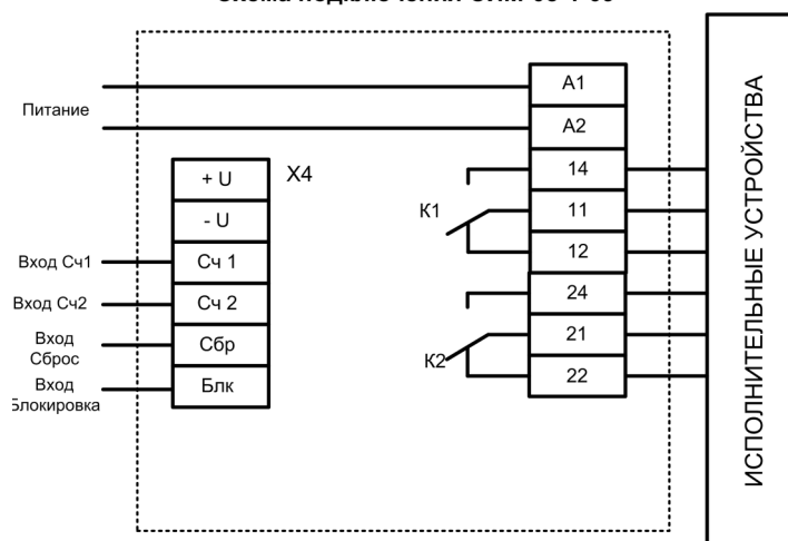
Схема подключения СИМ-05-1-09
